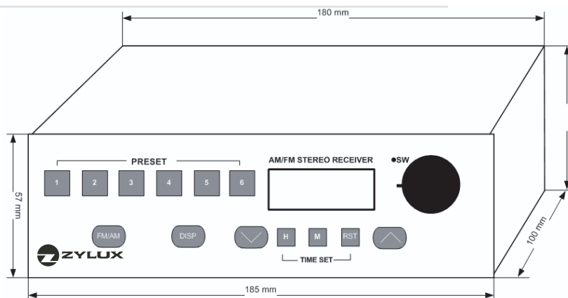
DIMENSIONS ZT-512 / ZT-524
